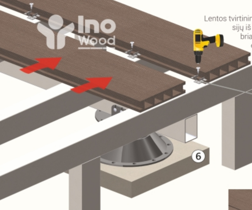
LENTOS TVIRTINIMO ELEMENTAS
